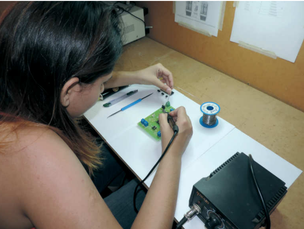
Montagem do Kit Mesh Solar: placa controla carga energética e permite a medição e o transporte, por rede, de dados sensoriais, como temperatura e níveis de luz
